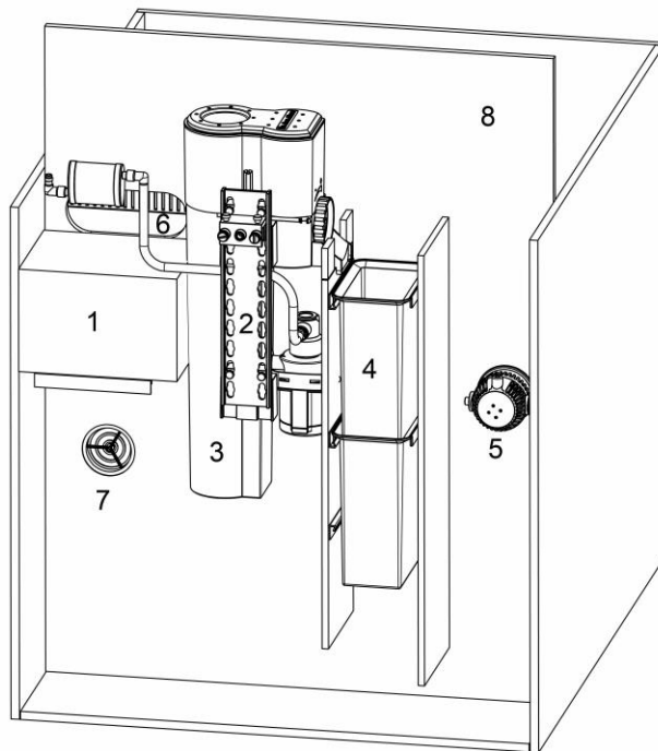
Fig. 1: Cámara de filtración de Cubicus Qube
